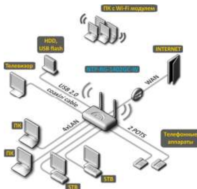
Рисунок 1 – Схема применения NTE-RG-1402
