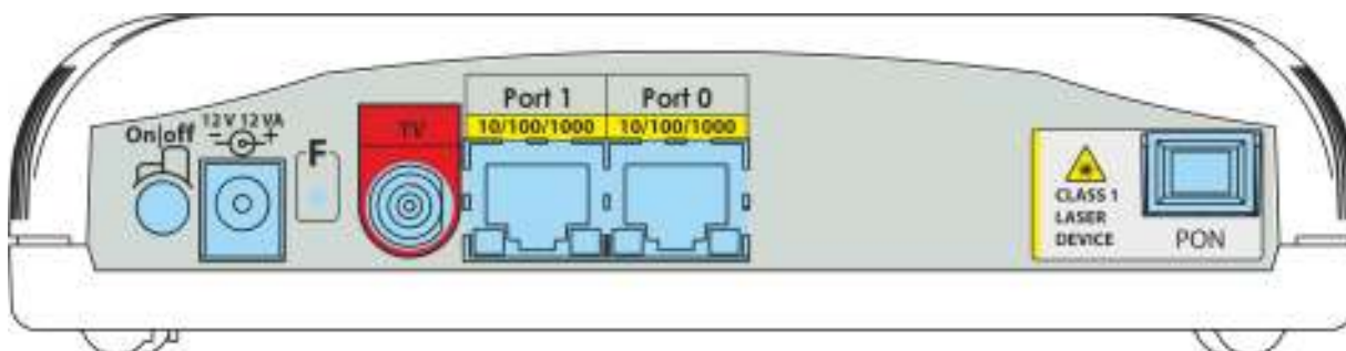
Рисунок 5 – Задняя панель абонентского терминала NTP-2C
