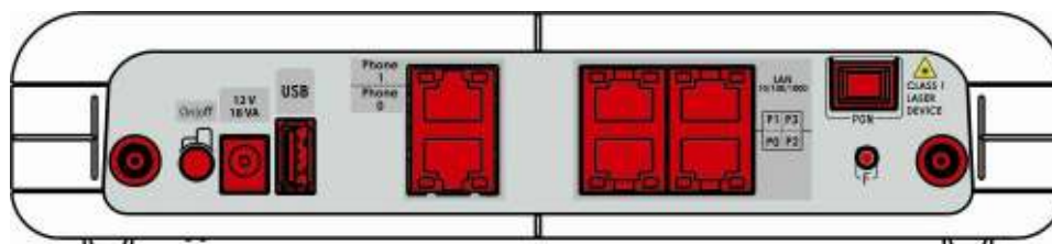
Рисунок 9 – Внешний вид задней панели NTP-RG-1402G-W
