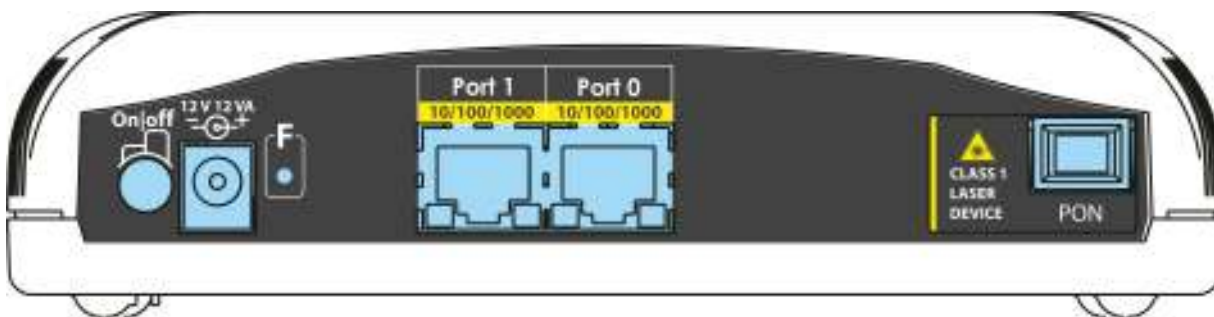
Рисунок 4 – Задняя панель абонентского терминала NTP-2
